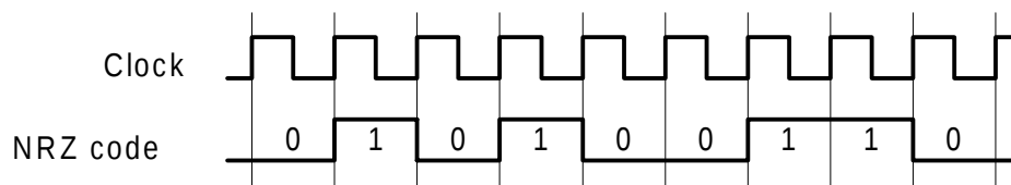
Fig. 3.1: NRZ code
